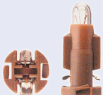
MF23 Long Life 12V 1,2W 203898 MF23 Long Life 12V 0,6W 203904
